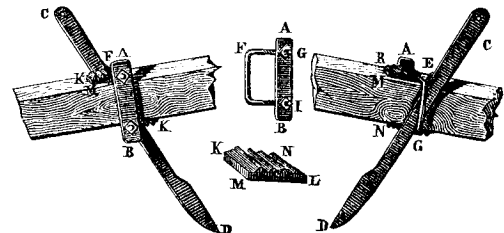
Fig. 3. 1° Haie de charrue armée d'un coutre CBD, maintenu par l'étrier américain ; 2° l'étrier FAB solé ; 3° plaque cannelée KNML ; 4° haie M armée d'un coutre CGD, vu entièrement.
